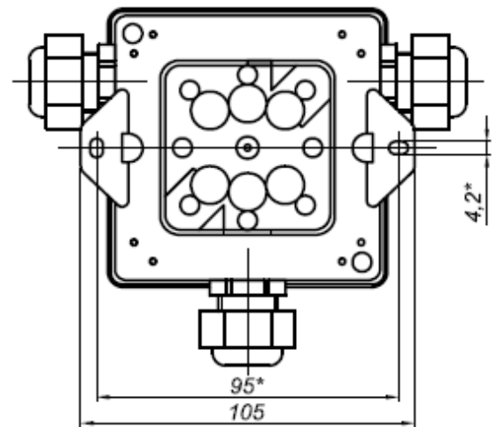
Вид А
